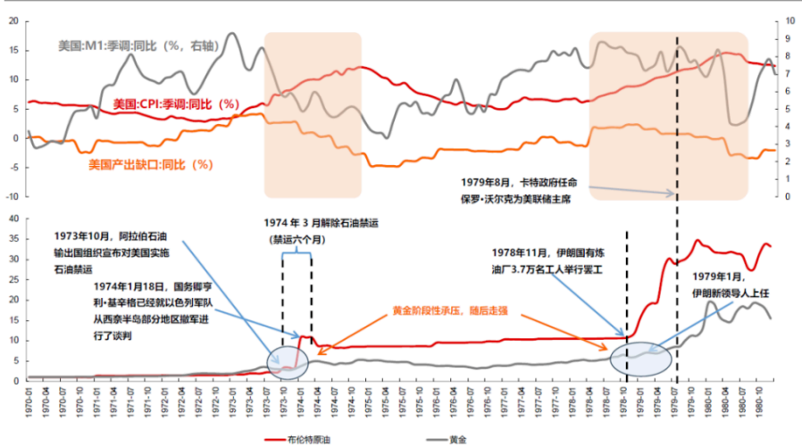
图 7：20 世纪两次石油危机来看，通胀上行叠加美国产出缺口回落阶段黄金表现显著占优，且战争初期黄金多受流动性冲击短暂承压，后续均迎来趋势性新高
